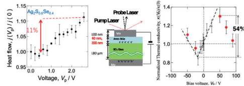
キャパシタ型熱流スイッチング素子の外観と性能
