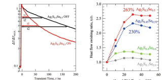
潜熱ポンプ型熱流スイッチング素子の性能
