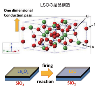
Reactive substrateとして石英ガラス基板を使用した基礎的研究を始め、基板上にc軸自己配向LSO薄膜が形成することを見出した。
