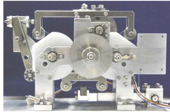
ワイヤソー切断装置の外観
