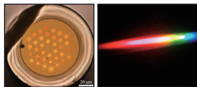
全固体微細構造光ファイバ 微細構造光ファイバからのスーパーコンティニューム光
